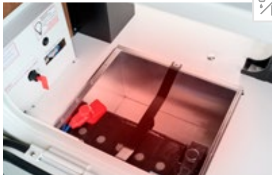
Batterisentral oppvarmet med batterihovedbryter. standard: 2 x 80 Ah gelbatterier, plassert lett tilgjengelig. Li-Ion-batteri som tilvalg, 90 Ah inkludert battericomputer.
