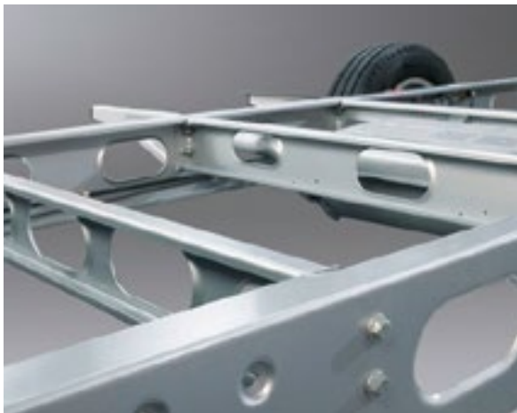
AL-KO lavramme spesial light
