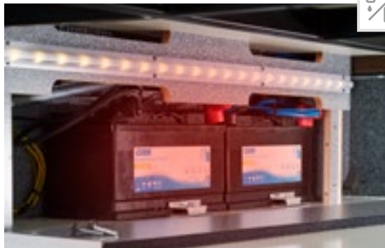
Standard batterisentral: 2 x 80 Ah gelbatterier i oppvarmet dobbeltgolv og batterihovedbryter. Li-Ion-batteri 90 Ah som tilvalg, inkludert battericomputer
