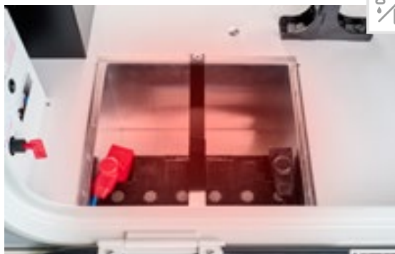
Oppvarmet batterisentral med batterihovedbryter. Standard: 1 x 80 Ah gelbatteri, kan utvides til 2 x 80 Ah. 90 Ah Li-Ion-batteri som tilvalg, inkludert battericomputer
